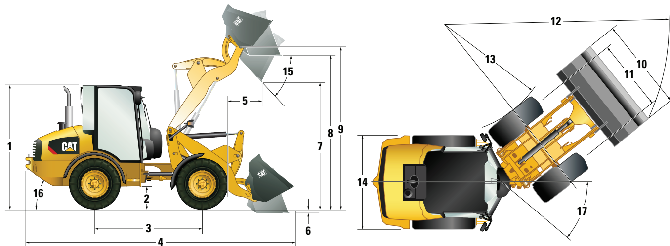
Standard-Hubgerüst – mit Kompaktlader-Schnellwechseleinrichtung
