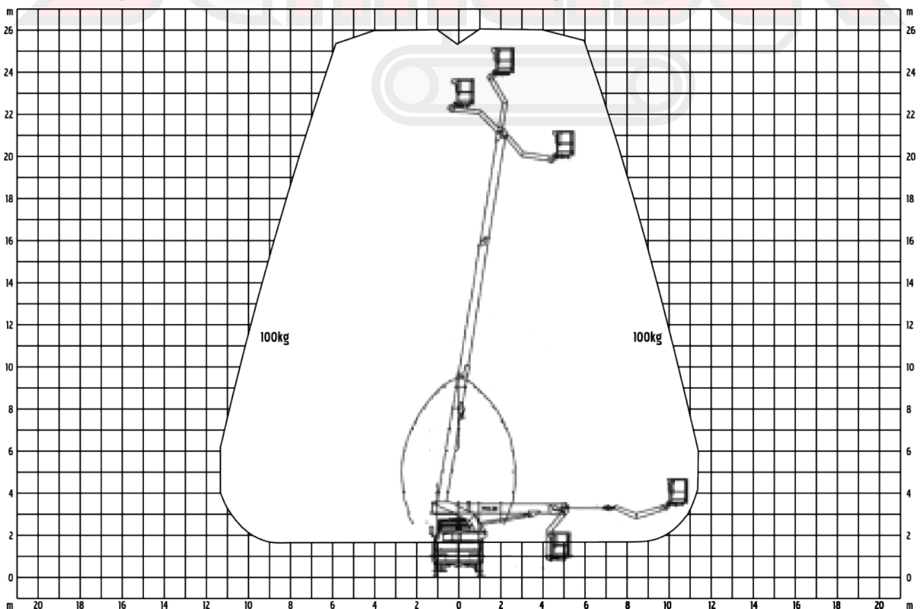
Reichweitendiagramm:
